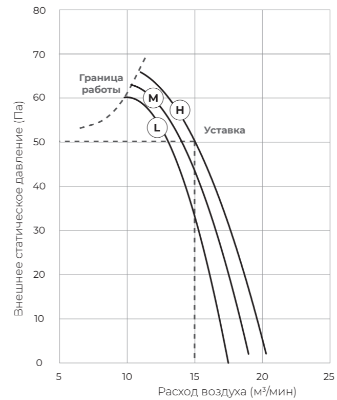
ADT-18UX4RCL8 (уставка 50 Па)
