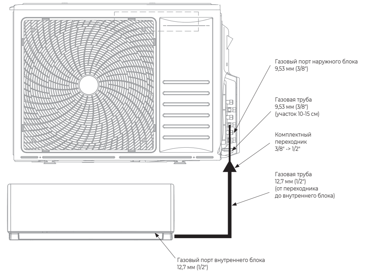
Образец выполнения соединения труб при несовпадении диаметра газовых труб наружного и внутреннего блока
